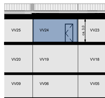
Doorsnede B-B
